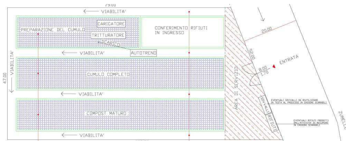
Layout dell'impianto
