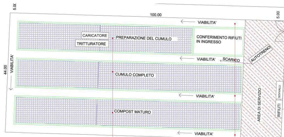
Layout dell'impianto
