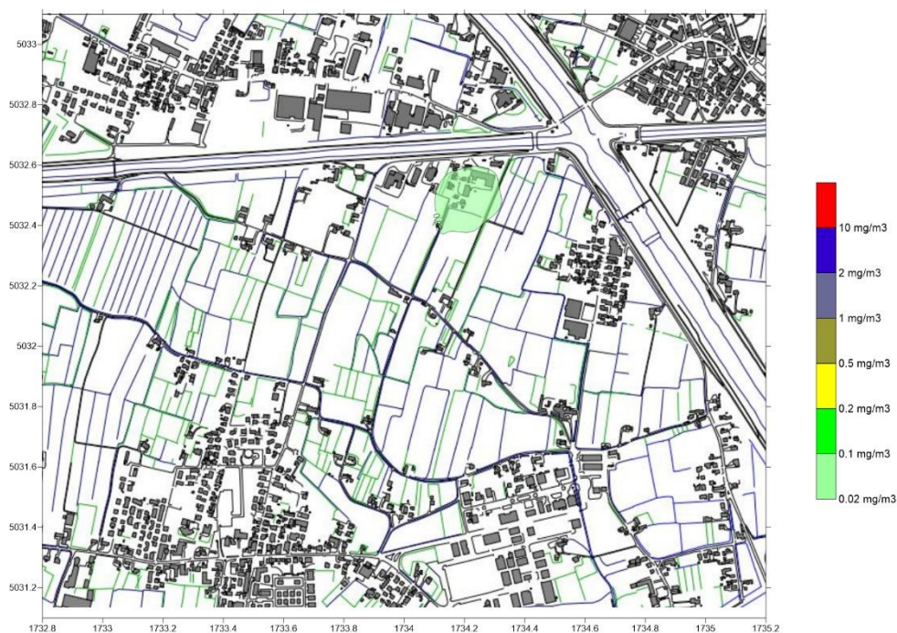
Figura 8 - Risultati della modellizzazione diffusionale. Concentrazione massima della media mobile giornaliera su 8 ore di CO. Scenario solo cogeneratore A
