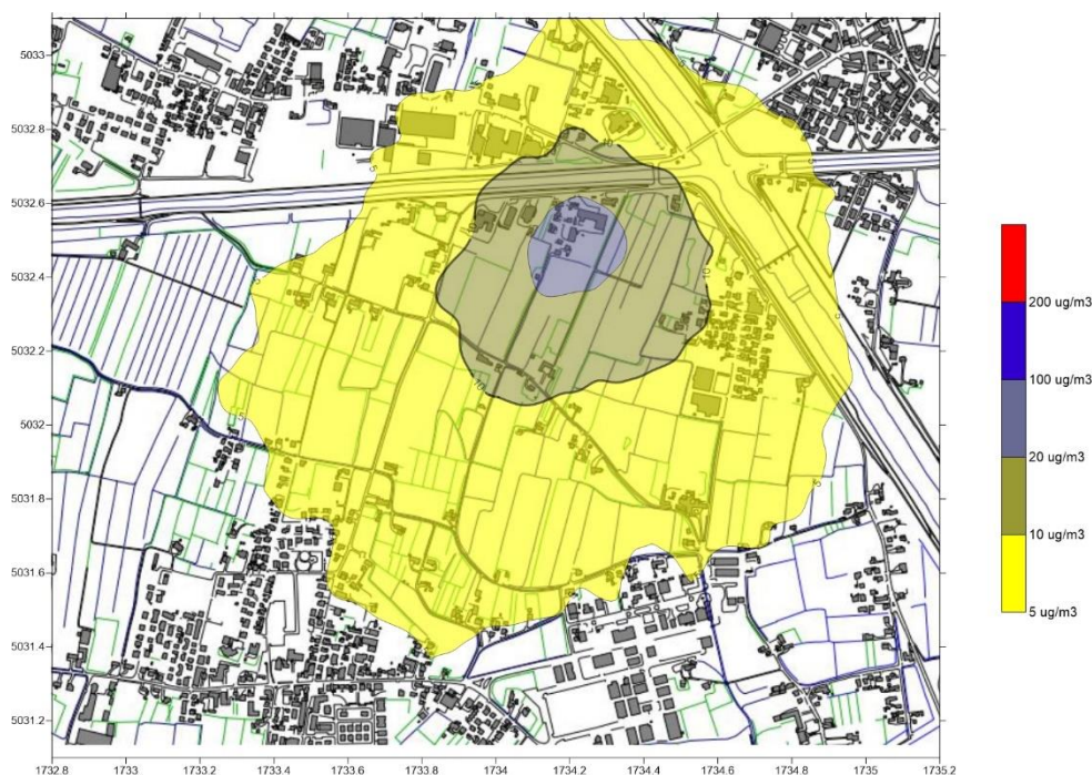
Figura 7 - Risultati della modellizzazione diffusionale. 19°esimo massimo annuo della concentrazione media oraria di NO2. Scenario cogeneratore A e B
