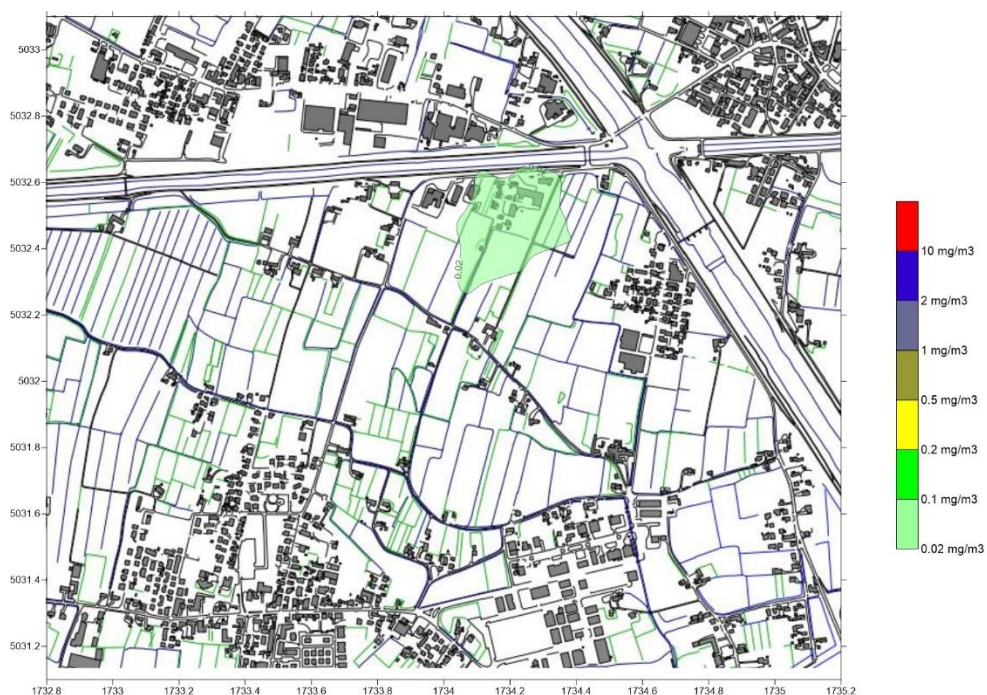
Figura 9 - Risultati della modellizzazione diffusionale. Concentrazione massima della media mobile giornaliera su 8 ore di CO. Scenario cogeneratori A e B
