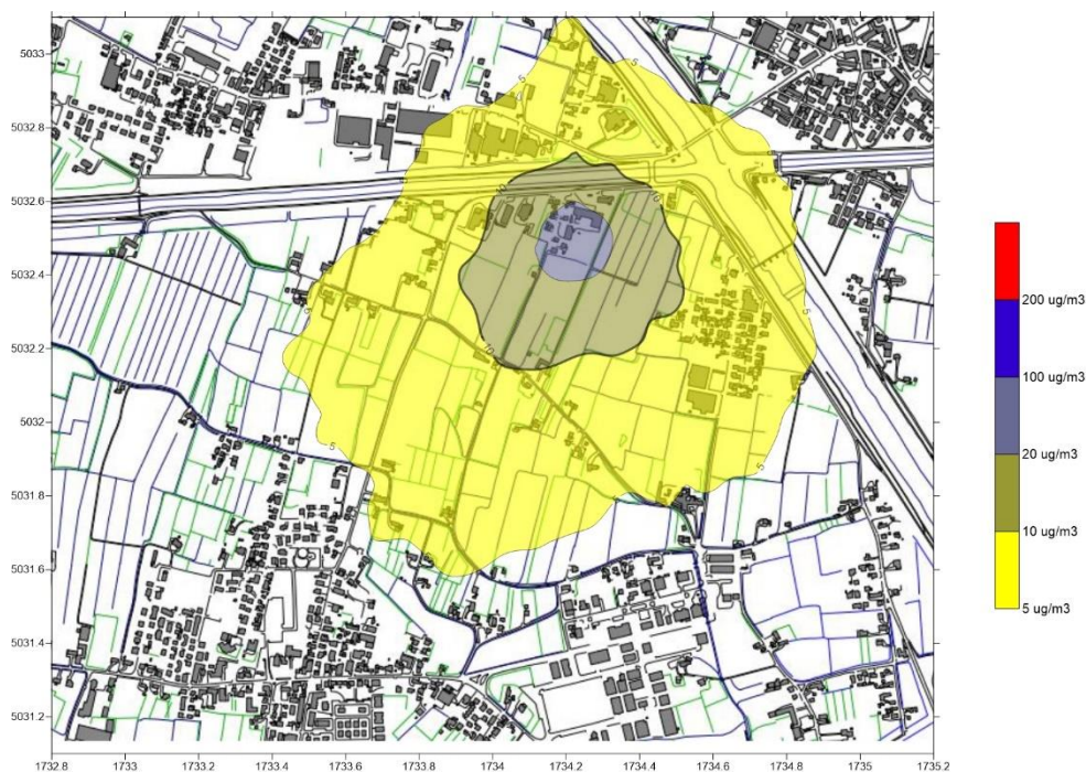
Figura 5 - Risultati della modellizzazione diffusionale. 10°esimo massimo annuo della concentrazione media oraria di NO2. Scenario solo cogeneratore A.
