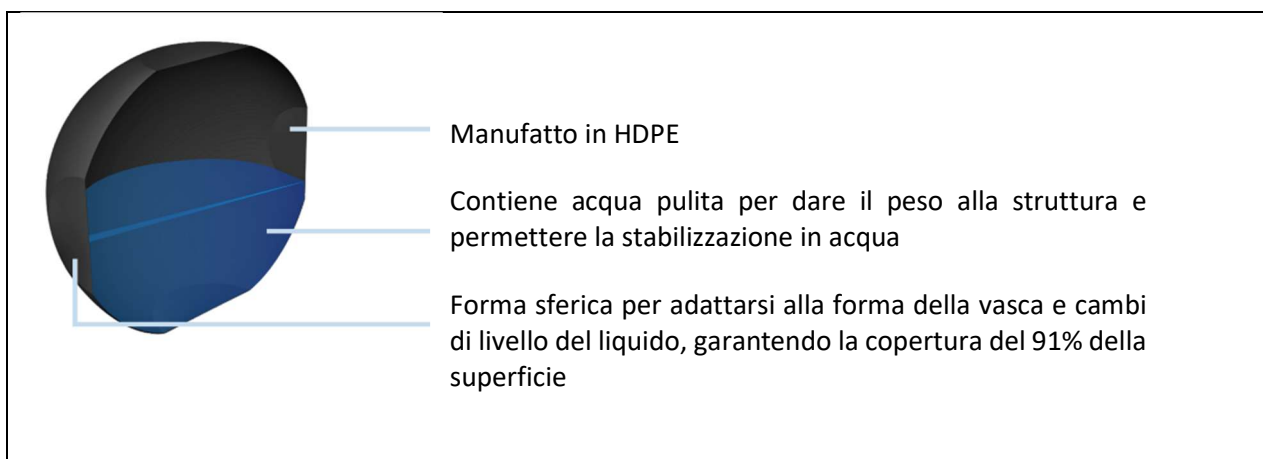
Figura 3: Caratteristiche della sfera galleggiante
