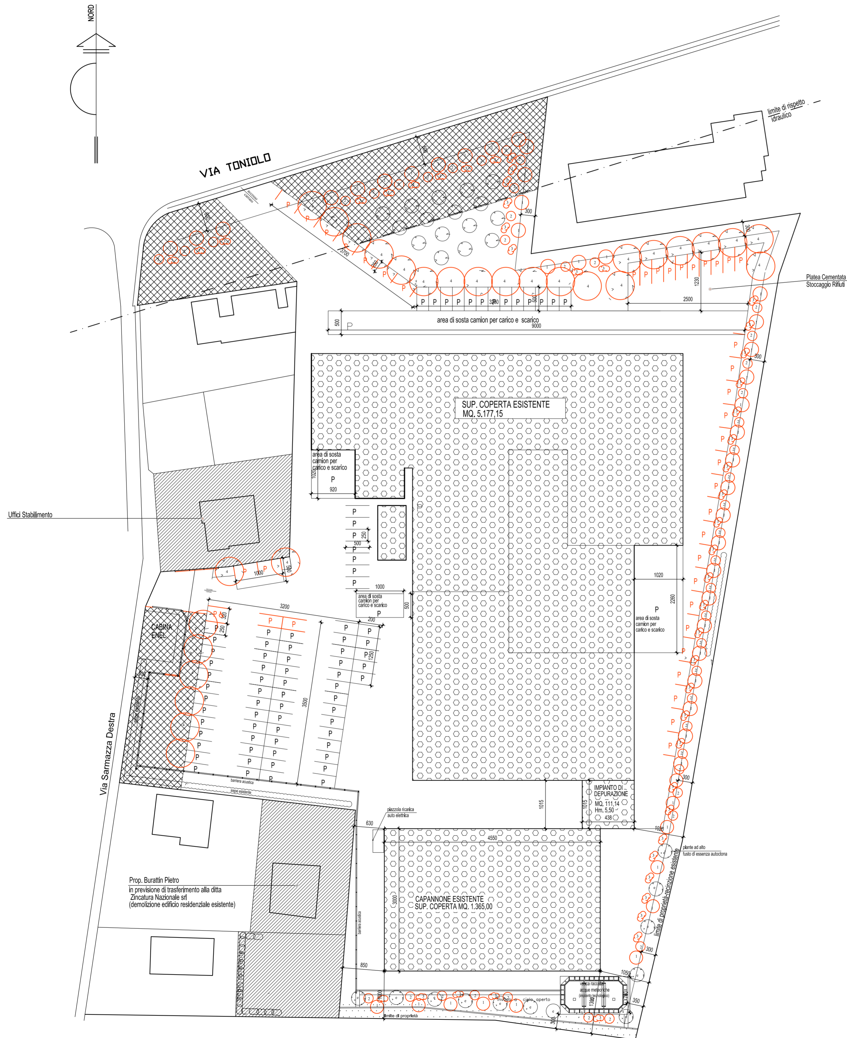
PLANIMETRIA di PROGETTO scala 1:500
